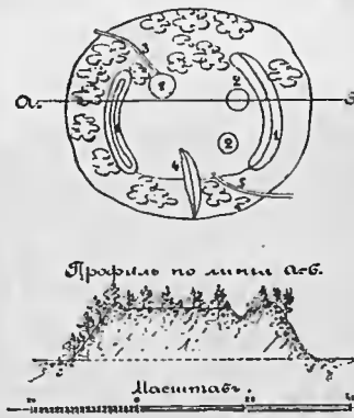
1 Остатки земл. валовъ. 2. Ямы, служившія порохов. хранилищами. 3. Тайниковая тропа. 4. Оврагъ, промытый водой. 5. Тропа, ведущая къ погосту.
